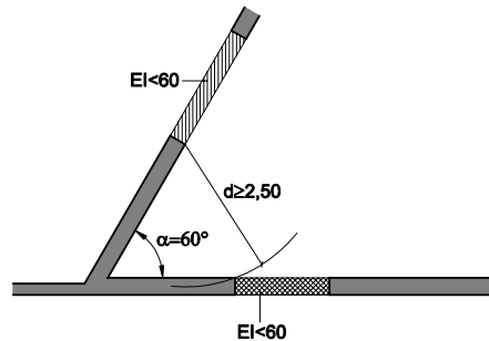
Figura 1.3. Fachadas a 60°
