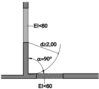
Figura 1.4. Fachadas a 90°
